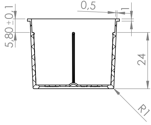
KESİT O-O
