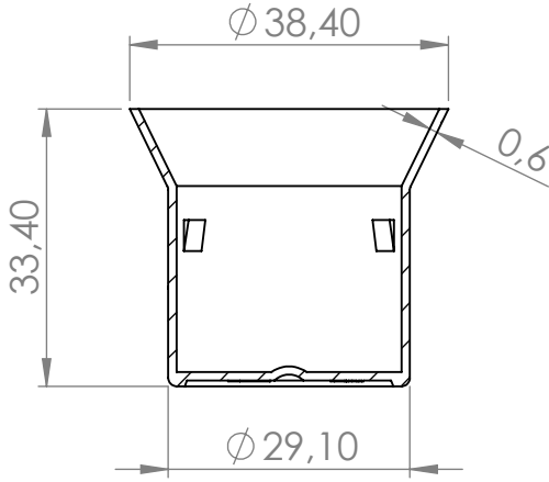
KESIT Q-Q
