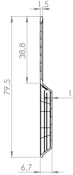
KESİT U-U
