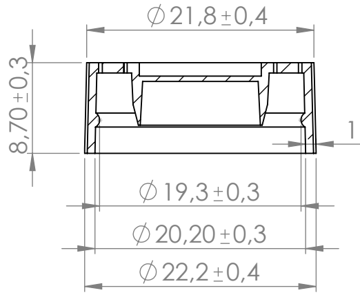
KESİT K-K
