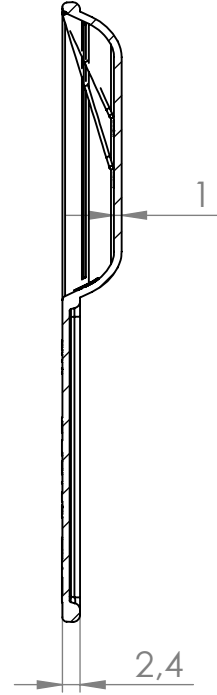
KESİT O-O
