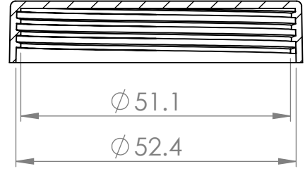
KESİT Q-Q
