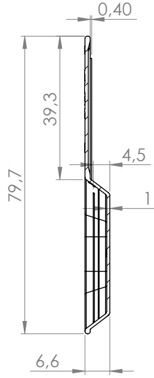
KESİT U-U
