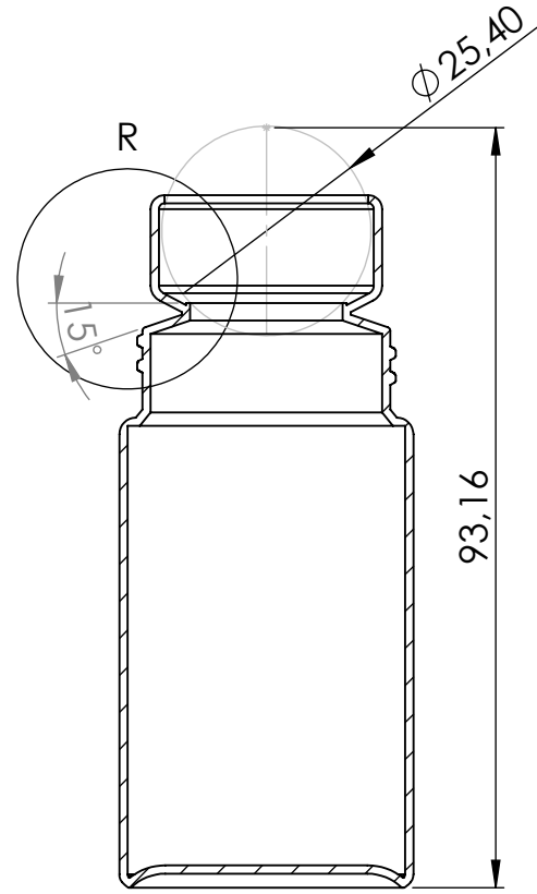
KESİT Q-Q ÖLÇEK 1 : 1
