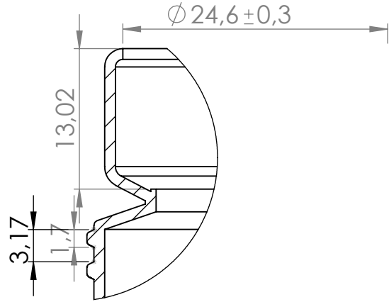
KESİT Q-Q ÖLÇEK 1 : 1
