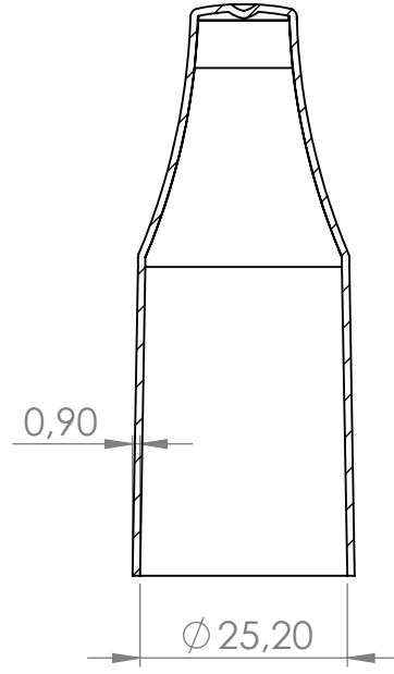
KESİT Q-Q
