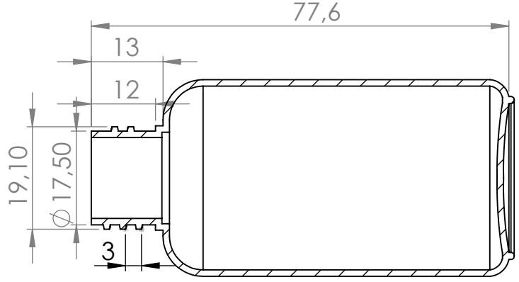
KESİT S-S ÖLÇEK 1 : 1
