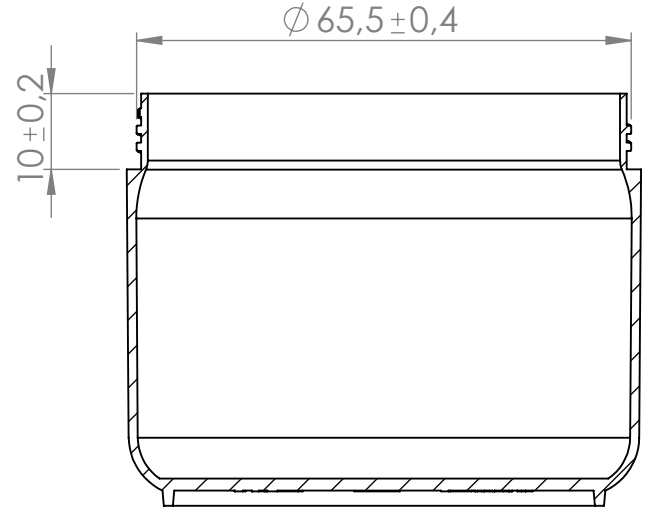
KESİT Q-Q ÖLÇEK 1 : 1
