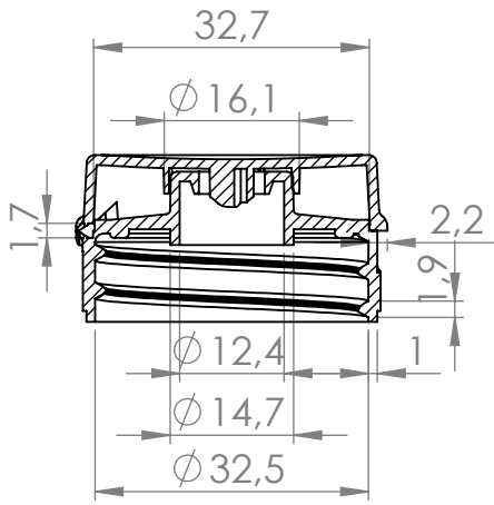
KESİT A-A
