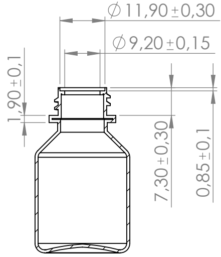
SECTION P-P SCALE 1 : 1
