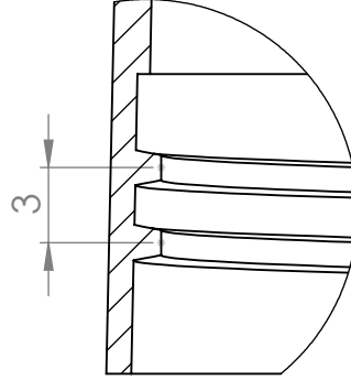
DETAY P ÖLÇEK 3 : 1
