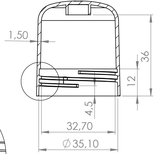
KESIT O-O
