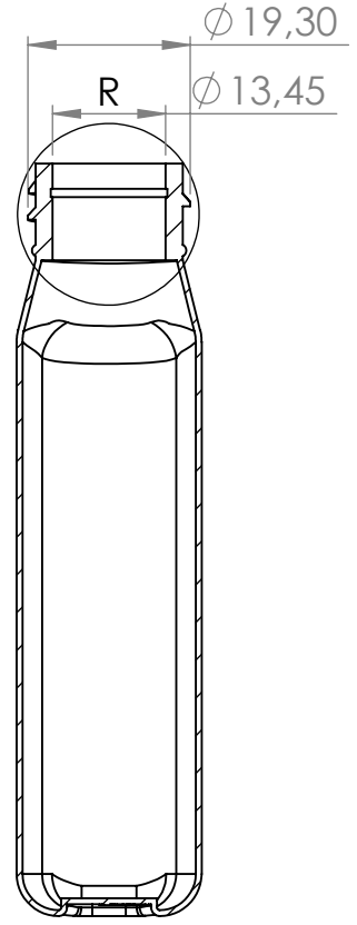
KESİT Q-Q ÖLÇEK 1 : 1
