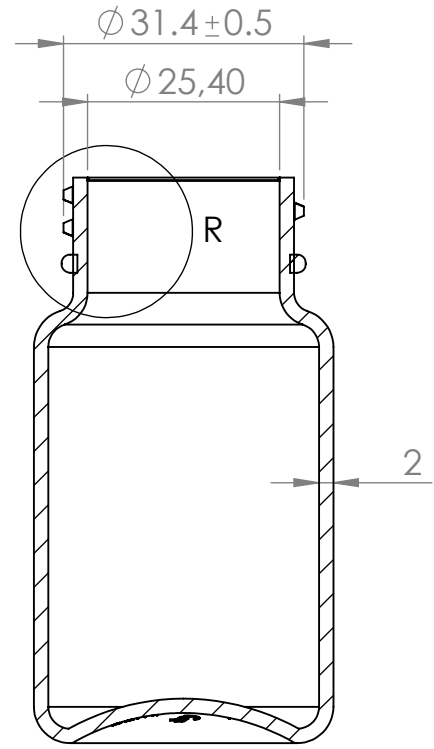
KESİT Q-Q
