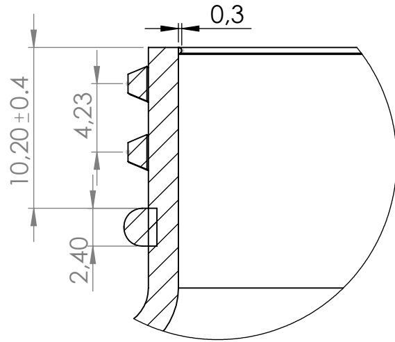
DETAY R ÖLÇEK 3 : 1
