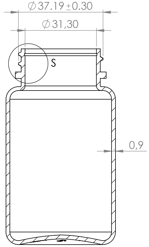
KESİT R-R
