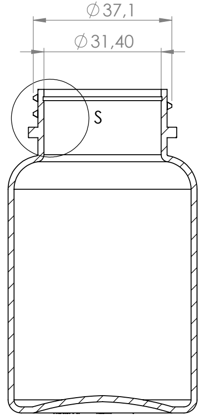
KESIT R-R
