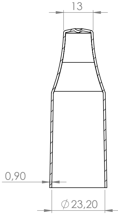
KESİT Q-Q
