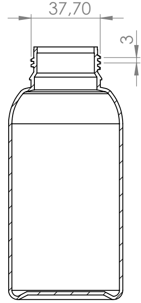
KESIT Q-Q
