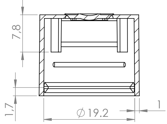
KESİT Q-Q
