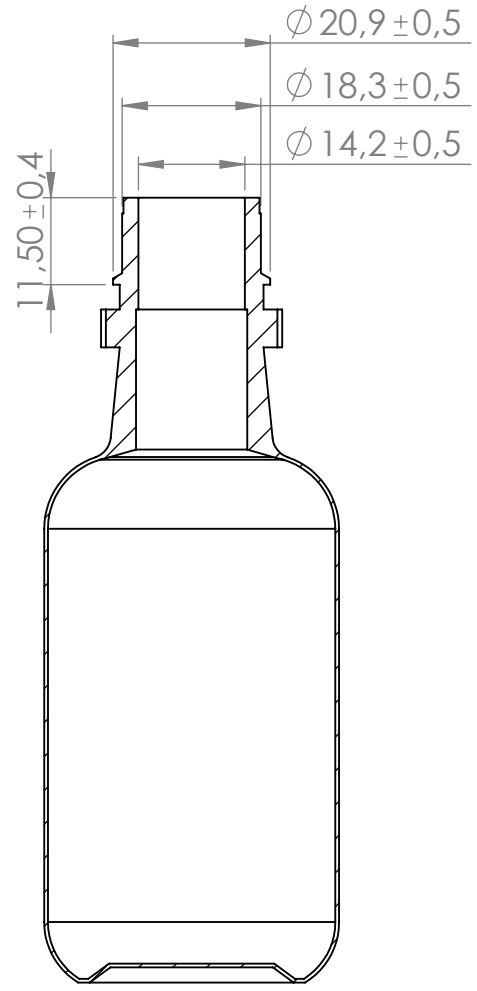
KESIT R-R
