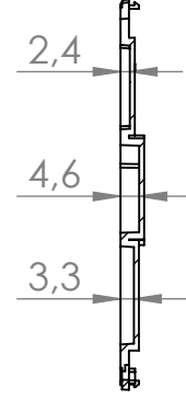
KESİT Q-Q ÖLÇEK 1 : 2
