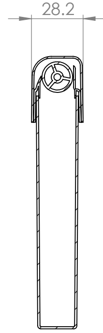
KESİT F-F ÖLÇEK 1 : 2
